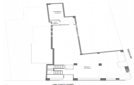
LOCAL COMERCIAL EN CALLE SANTA ISABEL ESQ. CALLE PLATERIA PLANTA BAJA PLANO DE DISTRIBUCIÓN / E.1:75 (DINA3)
